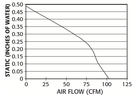
Fan Curve FV-08VQ2
